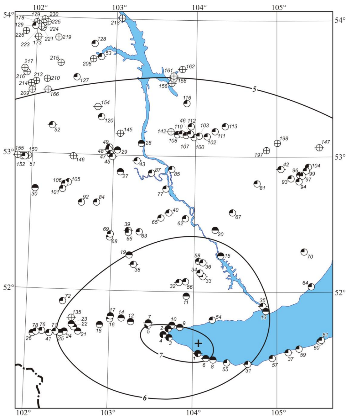
Рисунок 5. Схема макросейсмических проявлений землетрясения 27 авг. 2008 г. в 01 h 35 m в ближней зоне. Условные обозначения как на рисунке 4. Номера пунктов соответствуют таблице 1.
