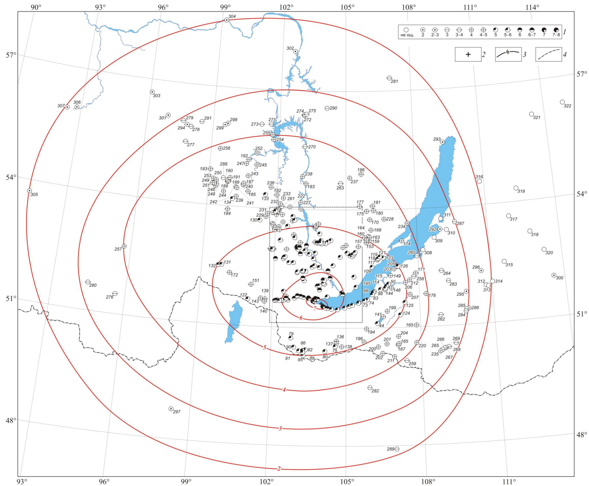
Рисунок 4. Схема макросейсмических проявлений землетрясения 27 авг. 2008 г. в 01 h 35 m .
